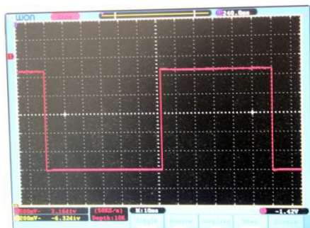
GN206W-P の短点波形
