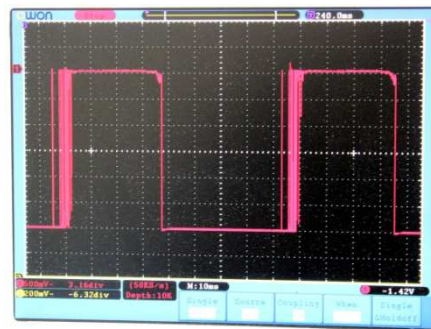
有名外国製バグキーの短点波形
